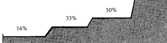
O.C.-Form BG1 – Exempel på tätningfunktion vid olika grader av komprimering i procent av ursprunglig tjocklek
